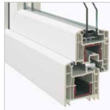
flächenversetzt | Anschlagdichtung
