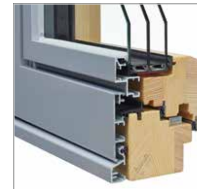
flächenbündig | Mitteldichtung
