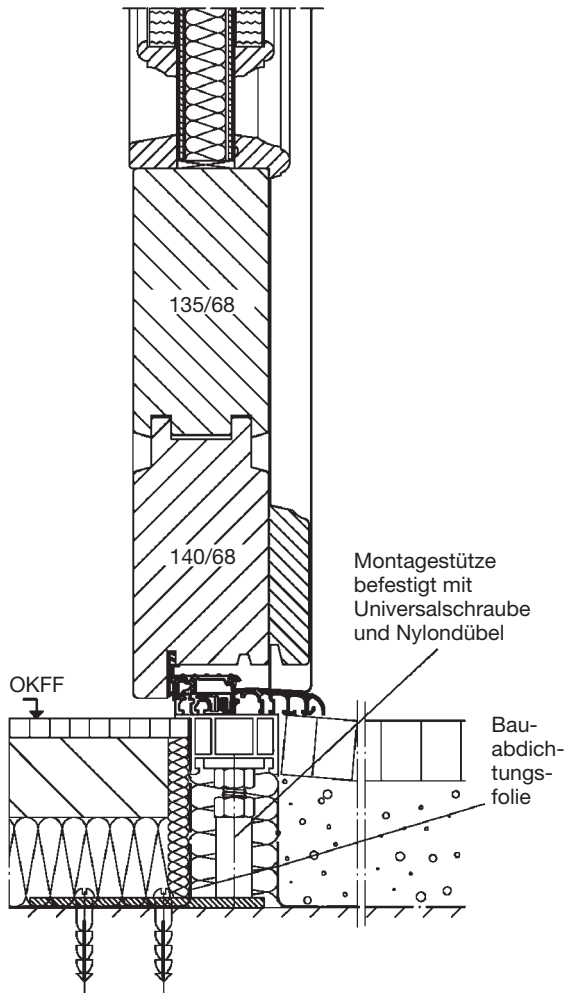
Unterer Anschluss Haustür
